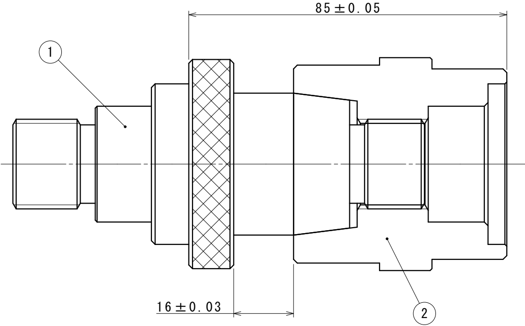
組立図A
