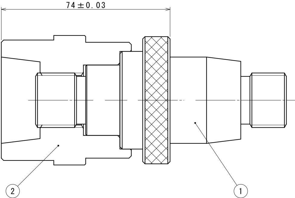
組立図B
